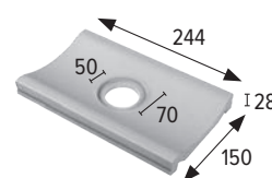
Canalina di trabocco con scarico Caniveau avec écoulement
