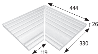
Griglia ceramica monocompact Grille céramique **
