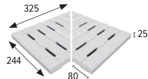
Angolo griglia Angle grille **
