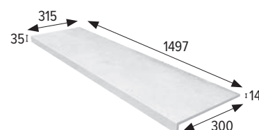
Bordo rettilineo 180* • Marche 180 * Disponibili a richiesta. / Disponibles sur commande.
