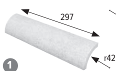
Angolo esterno 5 lati sguscio concavo Angle extérieur cornière
