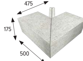
Pezzo angolare esterno Pièce angle extérieur
