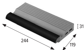
Angolo interno a 45° finlandese Angle intérieur onglet finlandais
