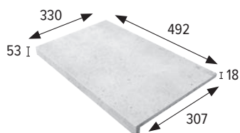
Bordo rettilineo 50 Marche 50
