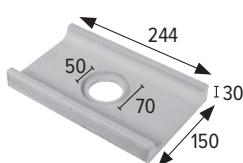
Canale con scarico Caniveau avec écoulement
