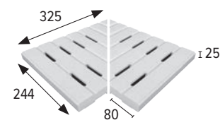
Angolo griglia Angle grille **
