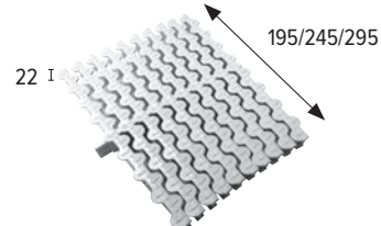
Griglia trasversale curva tipo F Grille transversale courbe type F
