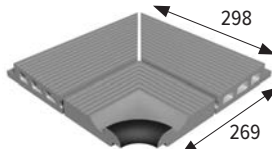
Angolo interno bordo GA SPA Angle intérieur bord GA-SPA
