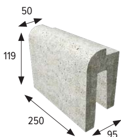
Pezzo arrotondato per mosaico Pièce arrondie pour mosaïque
