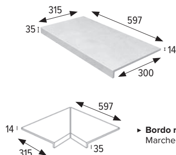
Bordo monocompact 120 • Bordure monocompact 120
