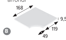
Angolo esterno arrotondato Angle intérieur bord arrondi
