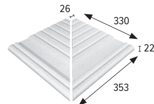
Angolo griglia Angle grille **
