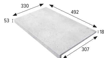
Bordo rettilineo 50 · Marche 50
