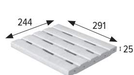
Griglia monocomp. scanalata Grille céramique rainurée**
