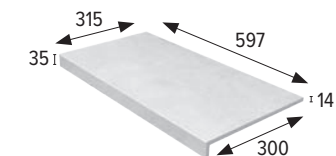
Bordo rettilineo 60 · Marche 60
