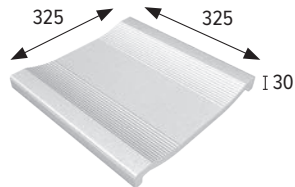
Canalina di trabocco Caniveau*
