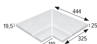
Angolo griglia Angle grille
