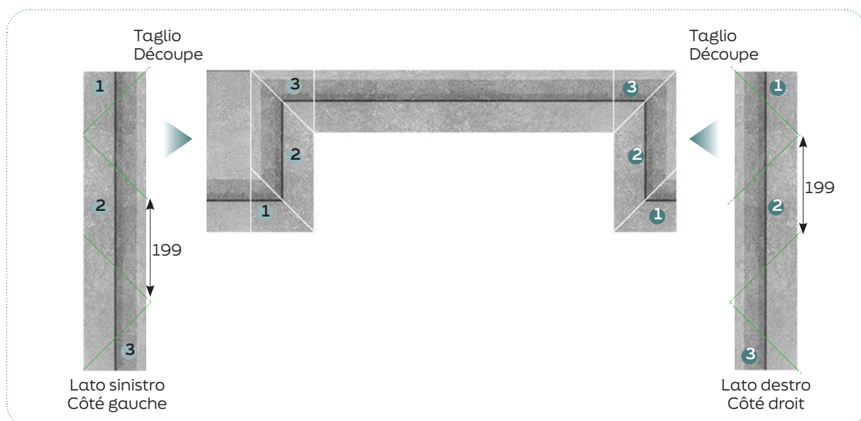
Pezzo nicchia con taglio bordo a sfioro 60 Pièce niche coupant bord débordant 60
