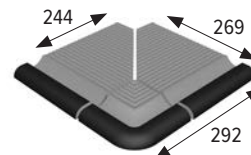
Angolo esterno bordo GA SPA Angle extérieur bord GA-SPA
