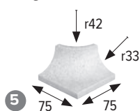
Angolo esterno 5 lati sguscio concavo Angle extérieur cornière
