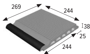
Nicchia GA-SPA Niche GA-SPA
