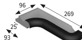
Angolo DX nicchia GA SPA Angle niche GA-SPA
