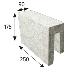
Pezzo nicchia Pièce niche
