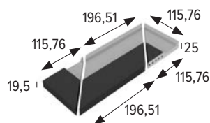
Angolo SX nicchia B33 SPORT Angle gauche niche B33 SPORT
