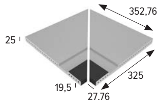
Angolo SX nicchia B33 SPORT Angle gauche niche B33 SPORT
