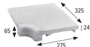
Rifinitura angolo interno Angle intérieur margelle
