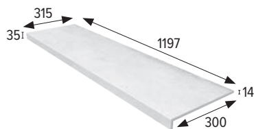
Bordo rettilineo 120 · Marche 120
