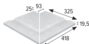
Griglia in ceramica a scomparsa Grille céramique cachée
